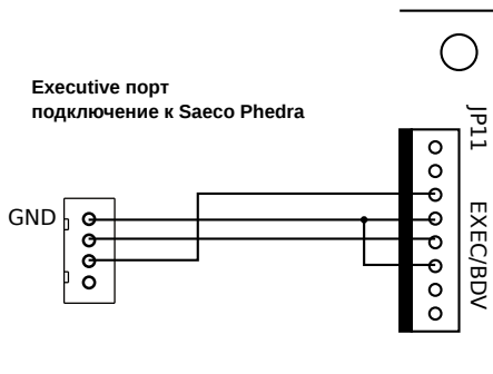
Saeco Phedra Разъем Exec/BDV вид на плату
