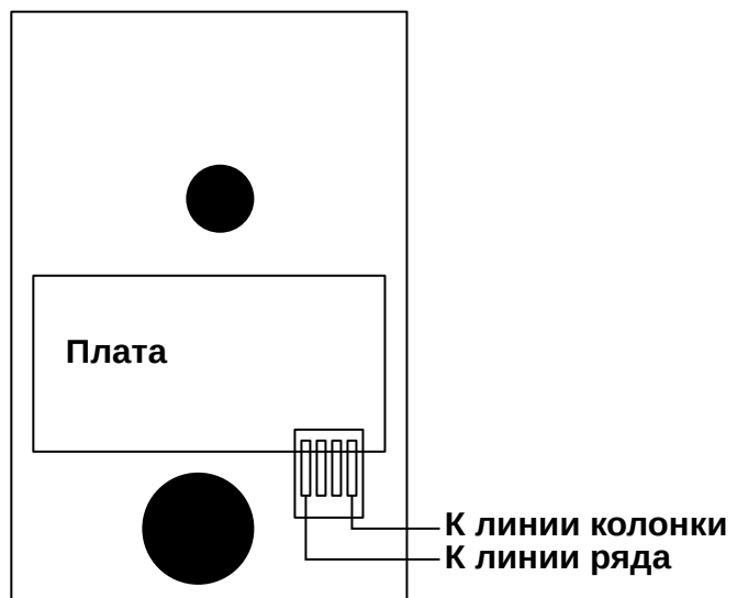
Привод спирали вид сзади
