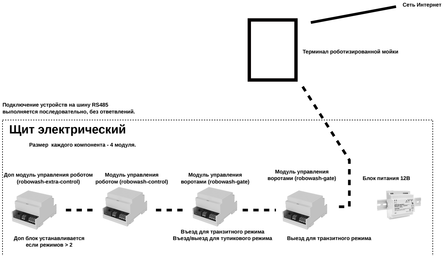
Модуль управления роботом (robowash-control)
