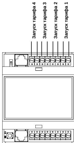
Модуль управления доп каналами робота (robowash-extra-control)
